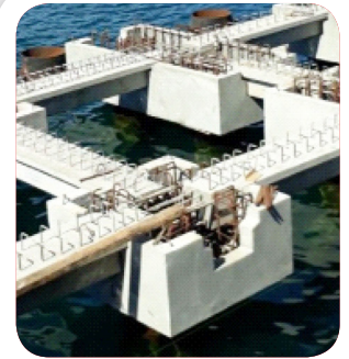
• Jetty Construction
