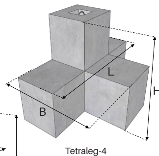
Tetrale-4
